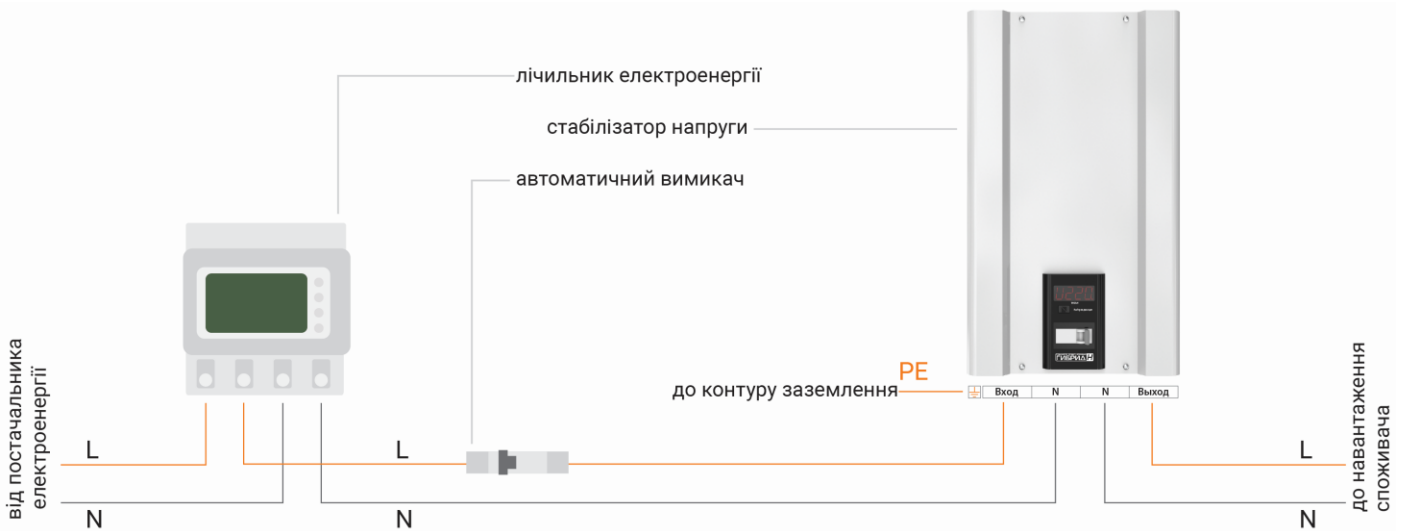
Рисунок 8. Схема підключення стабілізатора до однофазної мережі
