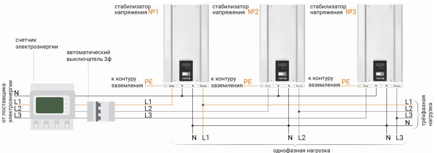
Рисунок 9. Схема подключения стабилизатора к трёхфазной сети
