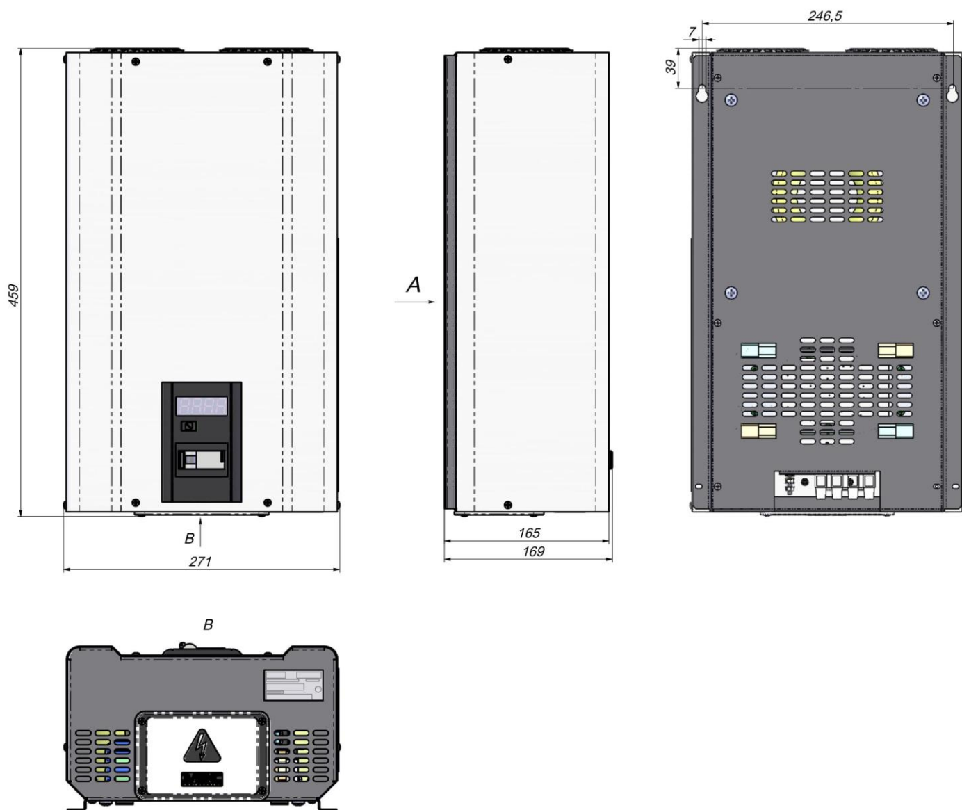
Рисунок 6. Габаритные и установочные размеры стабилизаторов ГИБРИД на 25, 32, 40А
