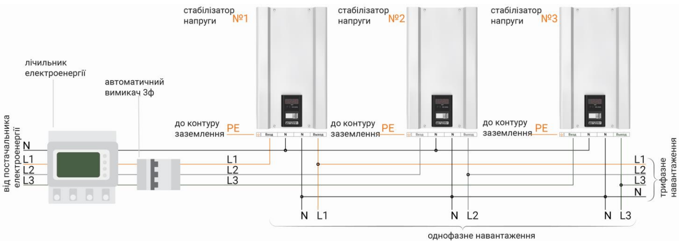
Рисунок 9. Схема підключення стабілізатора до трифазної мережі
