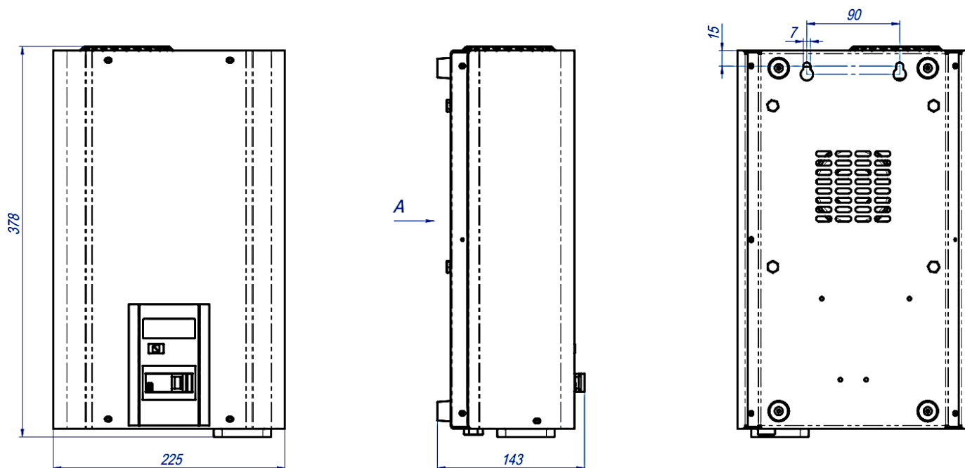
Рисунок 7. Габаритные и установочные размеры стабилизаторов ГИБРИД на 10 - 16А
