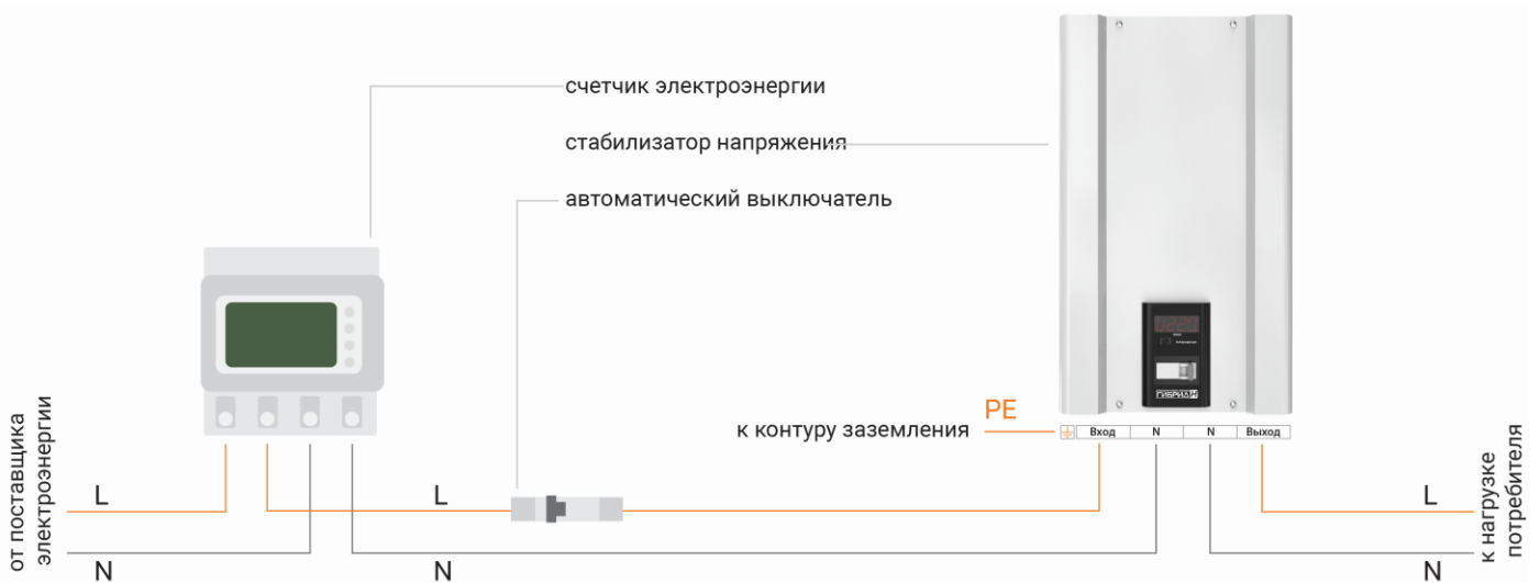
Рисунок 8. Схема подключения стабилизатора к однофазной сети
