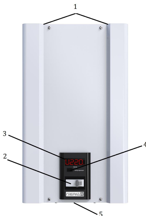
Рис.1 Внешний вид стабилизатора на 25-40А
