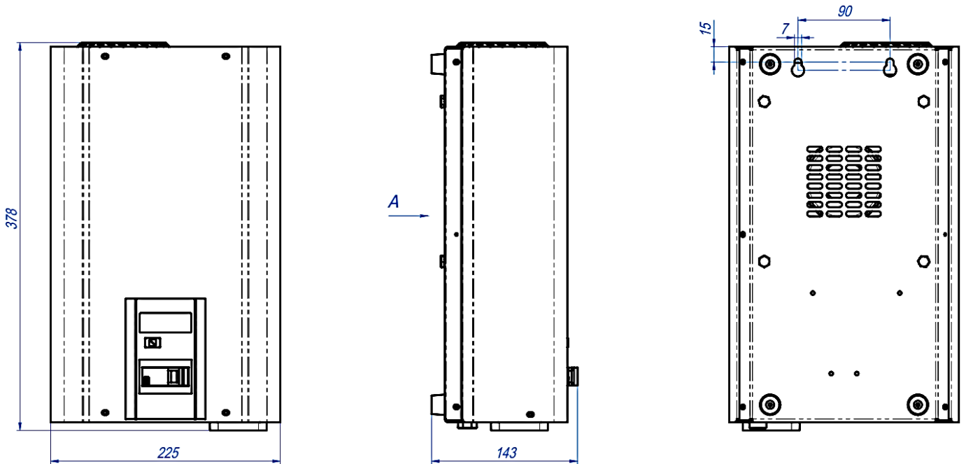
Рисунок 7. Габаритні та установочні розміри стабілізаторів ГБРИД на 10-16А
